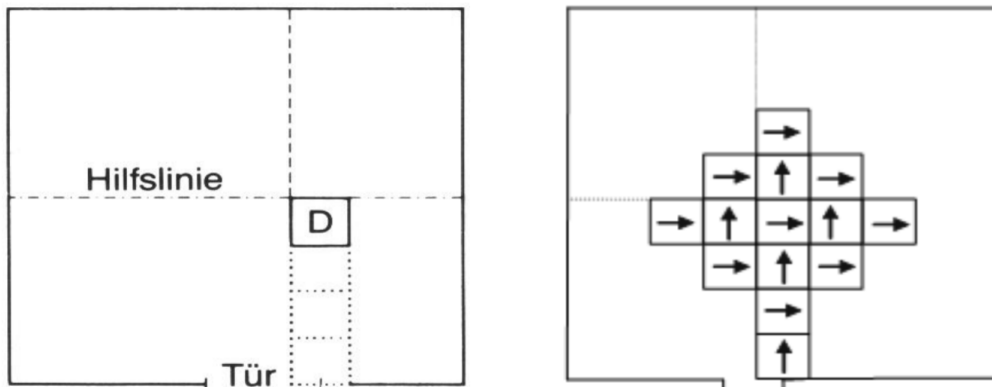
Anordnung der erste Fliesenreihe Parallel-/Schachbrett-Verlegung von Fliesen
